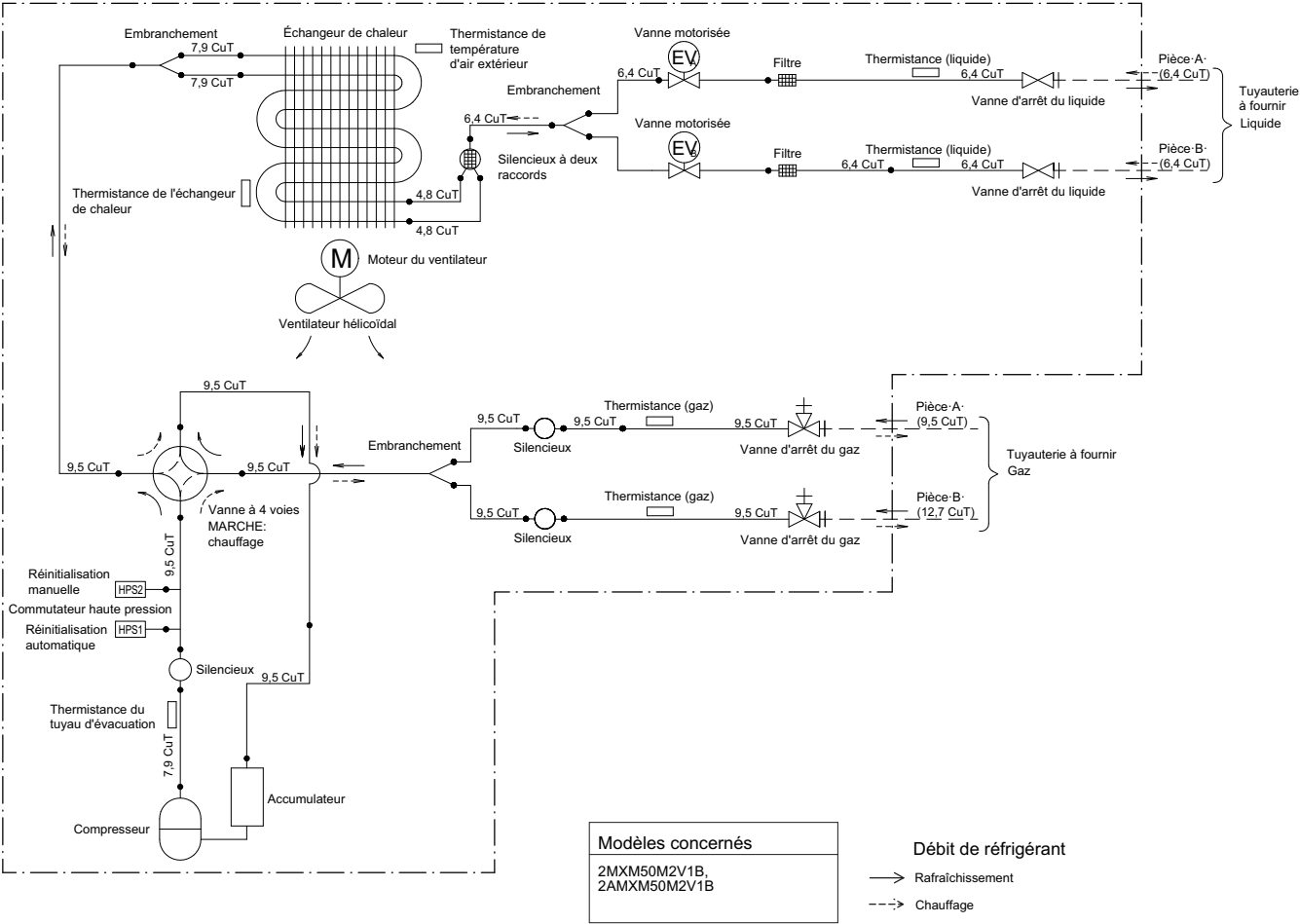
Unité extérieure
